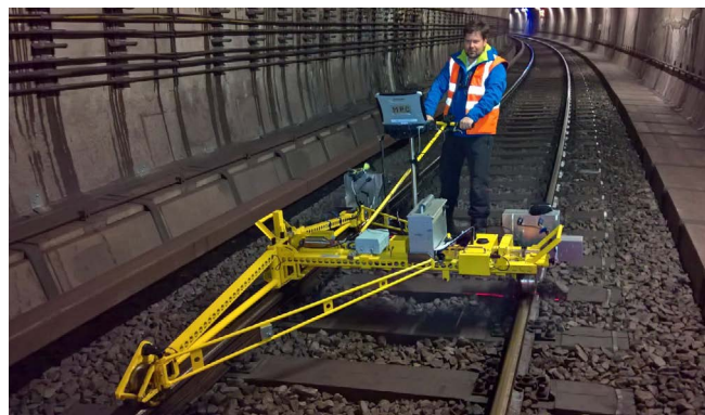
Mesure de la géométrie avec chariot KRAB
