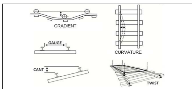
Paramètres de mesure de la voie : Gradient, écartement, dévers, courbe, torsion
