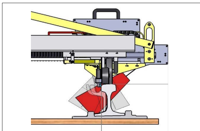
3 lasers par rail pour les mesures du champignon des rails à gorge et des rails Vignole
