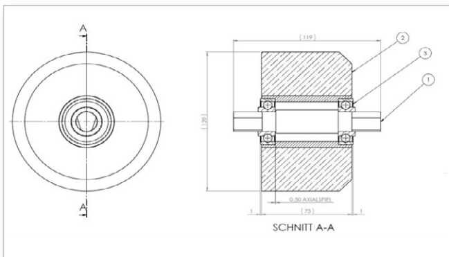
Fahrkanten-Schleifkörper
