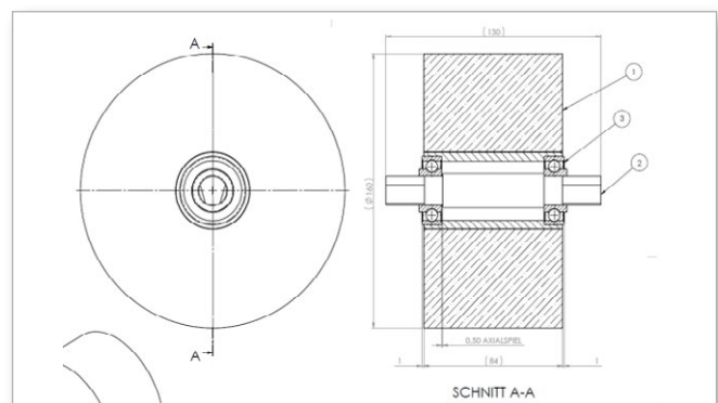
Fahrflächen-Schleifkörper
