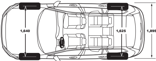
●日本仕様は右ハンドルのみの設定となります。 単位：mm
